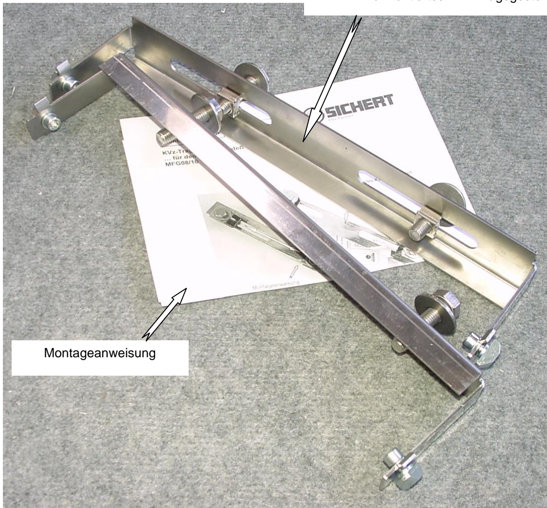
vormontiertes KVz-Tragegestell
